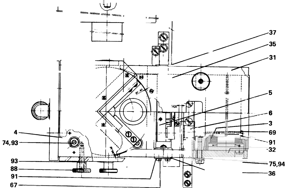
Electron beam evaporation source / Elektronenstrahl-Verdampfungsquelle ESQ 113 BB 800 059 E/1 BB 800 059 E/2
